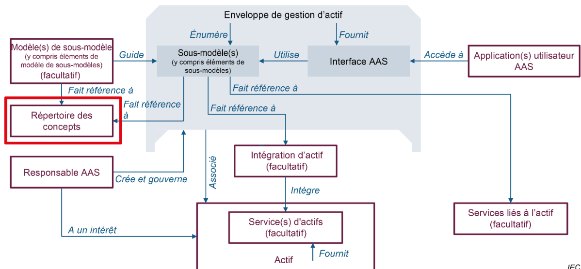
Figure 1 – Vue d'ensemble détaillée de l'enveloppe de gestion d'actif et entités connexes (d'après l'IEC 63278-1)
